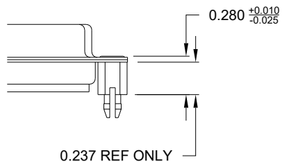
"92" // PCB SIDE **
